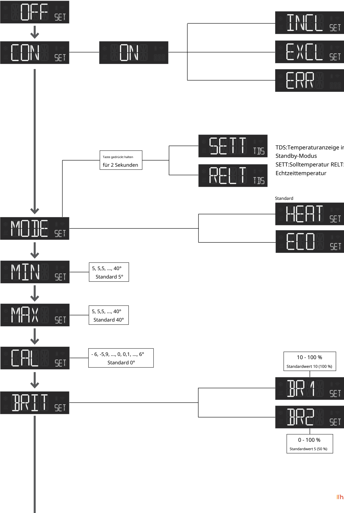
28. DIAGRAMM - ANZEIGEMENÜSTRUKTUR Halten Sie die mittlere Taste 5 Sekunden lang gedrückt, um ins Menü zu gelangen.
